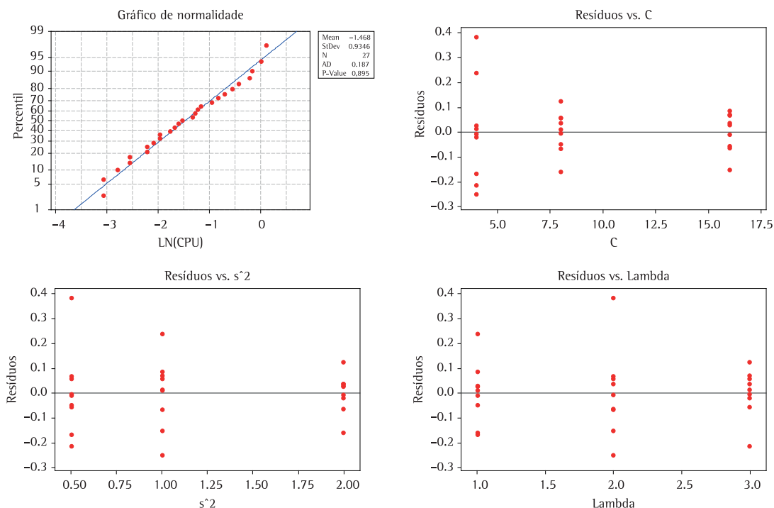
Figura 7. Suposições iniciais do modelo proposto para análise de desempenho. Fonte: MINITAB 15.
