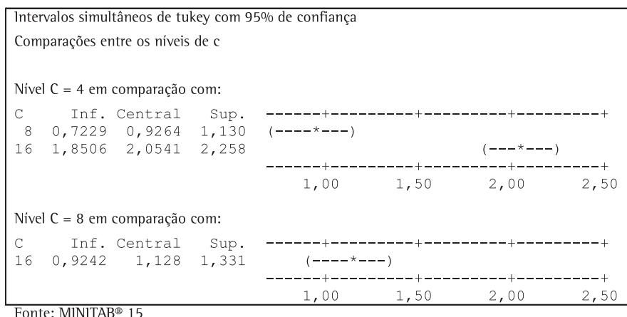
Figura 5. Comparações múltiplas entre os níveis do número de servidores. Fonte: MINITAB 15.
